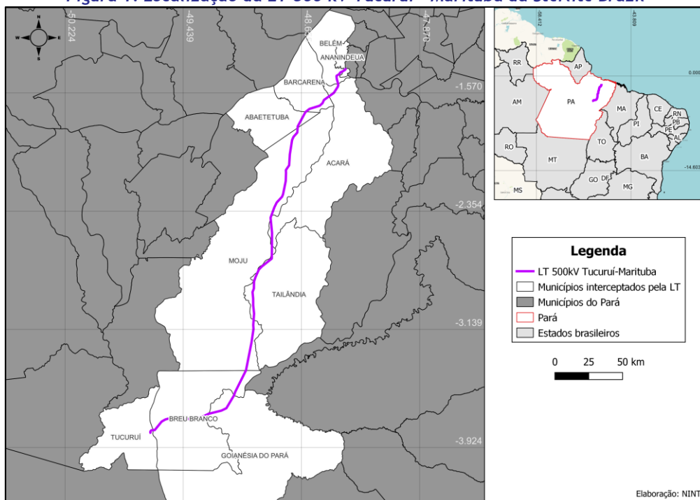
Figura 1. Localização da LT 500 kV Tucuruí - Marituba da Sterlite Brazil
